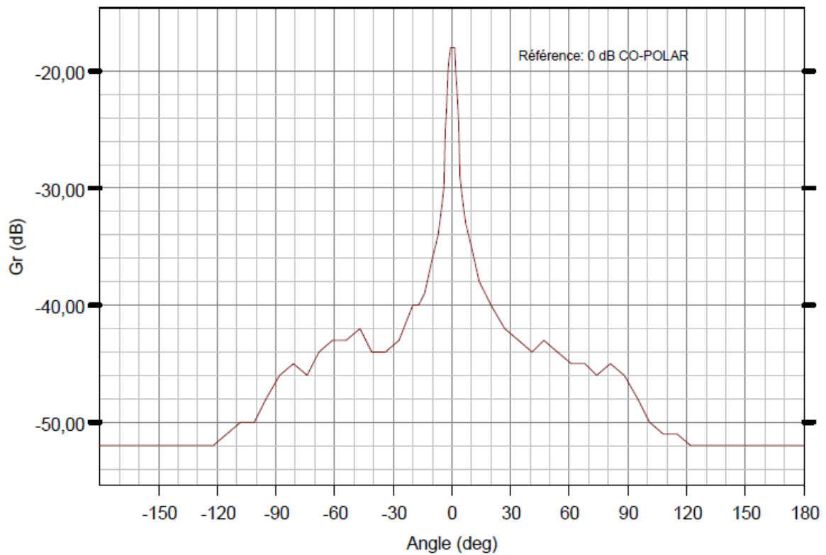
Antenne parabolique 63 cm avec radôme - CR
