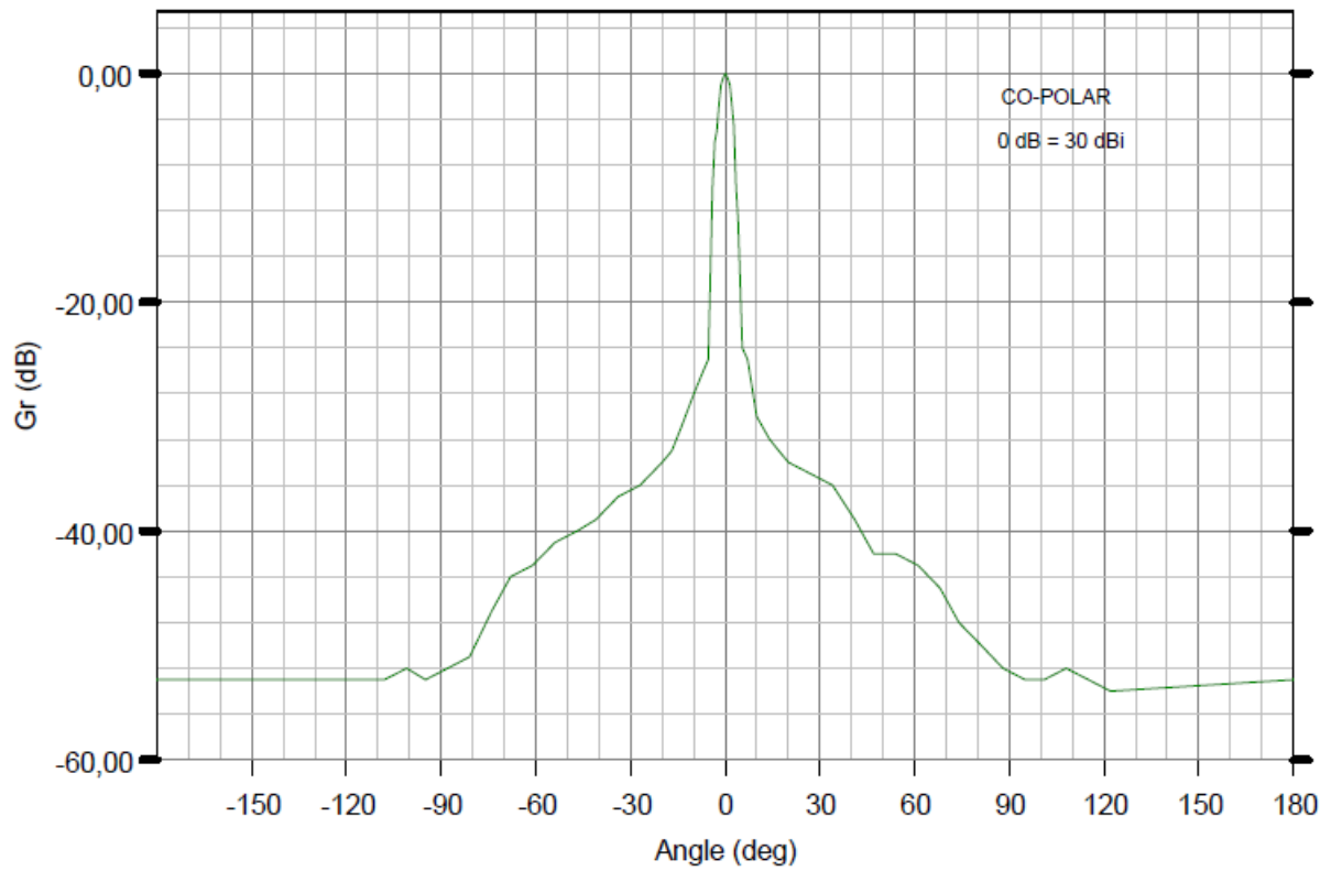
Antenne parabolique 63 cm avec radôme - CR
